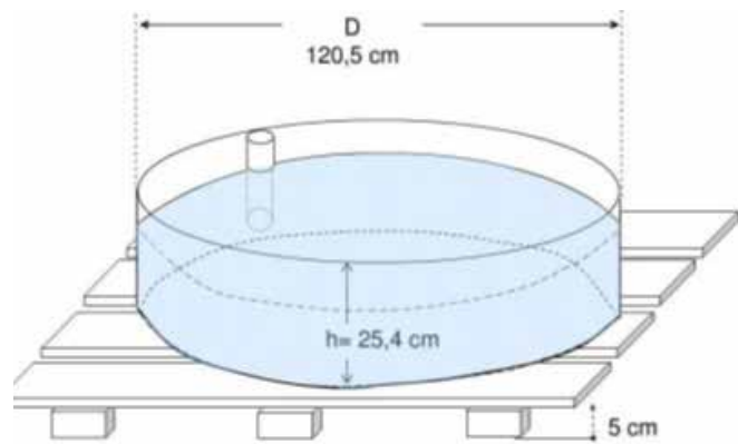
Modelo del tanque evaporímetro clase A. Fuente: Universidad Nacional De Colombia
