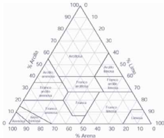
Triángulo de texturas. Fuente: USDA
