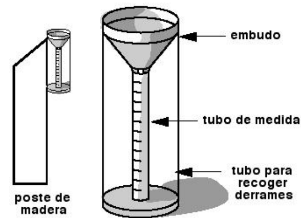
Pluviómetro para medir precipitación. Fuente: itsamexico.com
