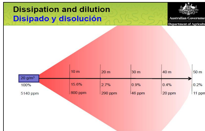
Figura 28 Gráfico que muestra la disipación y dilución del bromuro de metilo al momento de la aereación. Nota: Manual de Fumigación con bromuro de metilo según Norma de la DAFF
