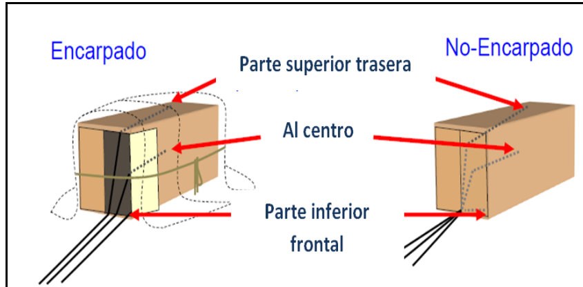
Figura 20 Esquemas de distribución de sondas de monitoreo en contenedores. Nota: Manual de Fumigación con bromuro de metilo según la Norma de la DAFF
