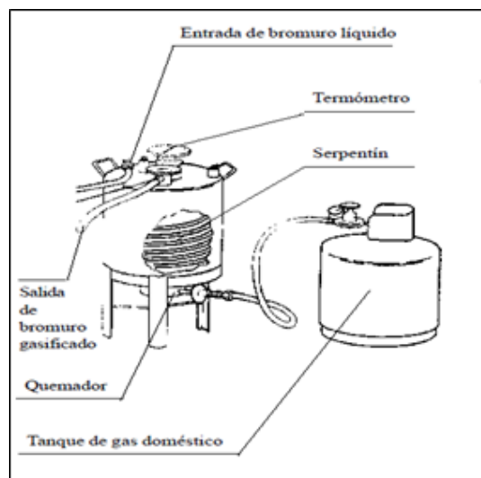
Imagen 13 Esquema de las partes de vaporizador para aplicación de bromuro de metilo
