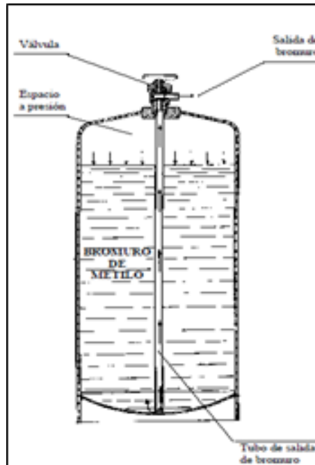
Figura 9 Esquema del cilindro de bromuro de metilo.
