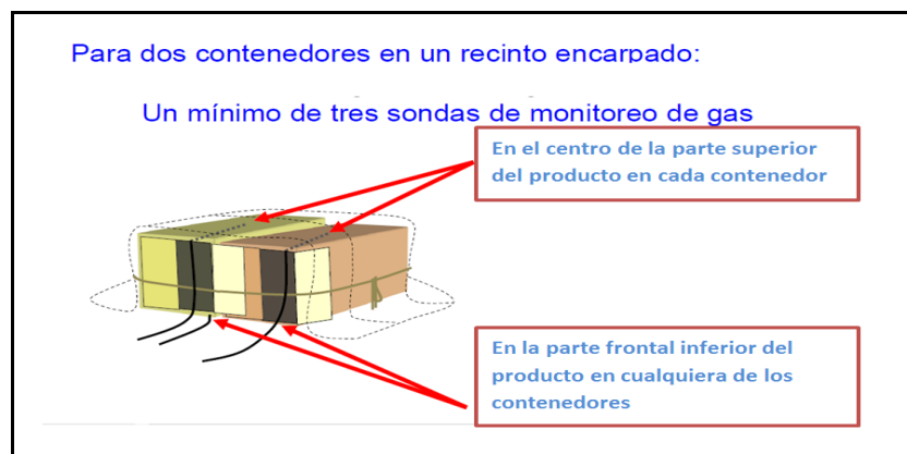
Figura 21 Distribución de sondas de monitoreo en recintos encarpados. Nota: Manual de Fumigación con bromuro de metilo según la Norma de la DAFF
