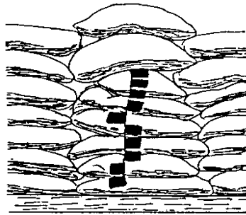
Figura 4 Esquema de como colocar las bosas, sachets o cadenas con fosfina con respecto a la mercadería
