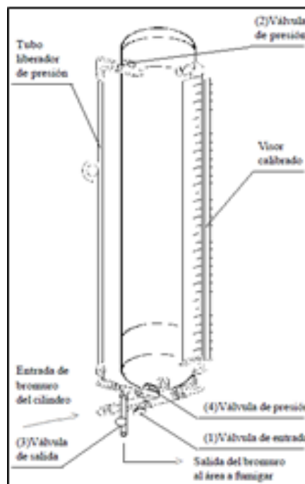
Figura 11 Esquema del dosificador para bromuro de metilo.
